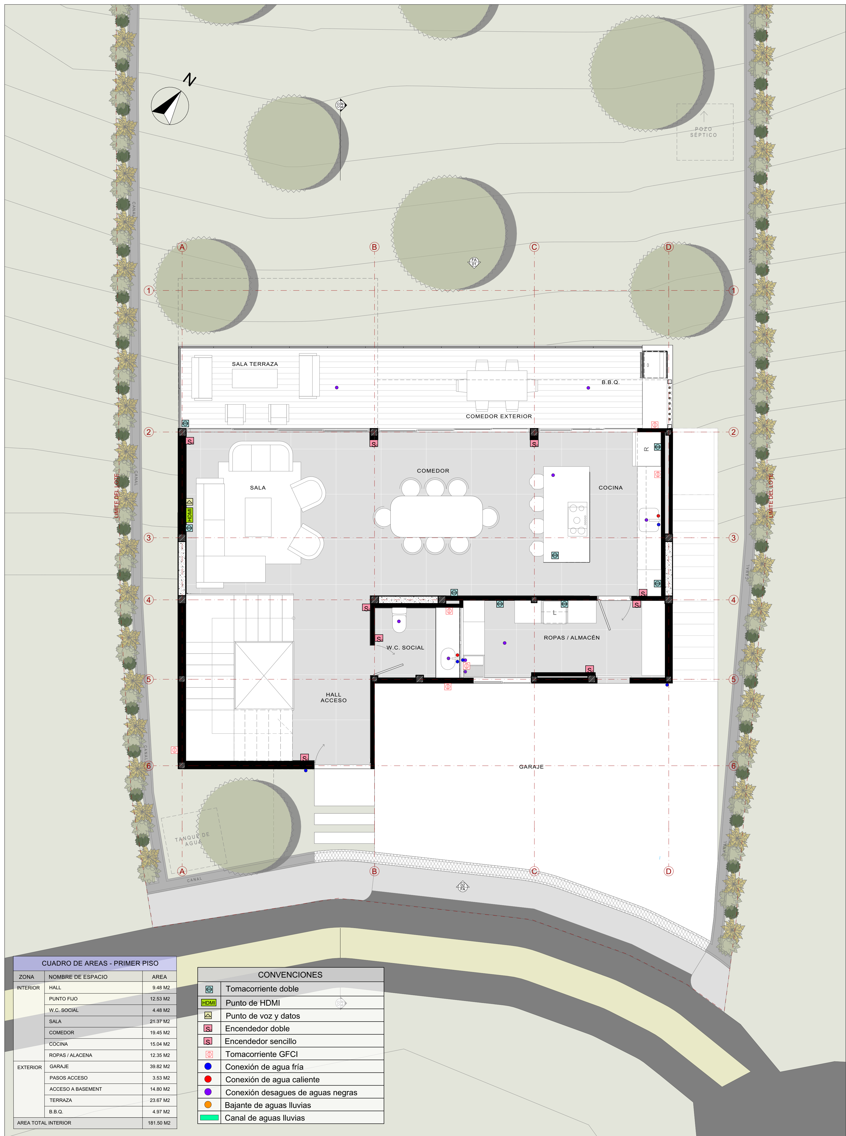
Plano de Primer Piso:
