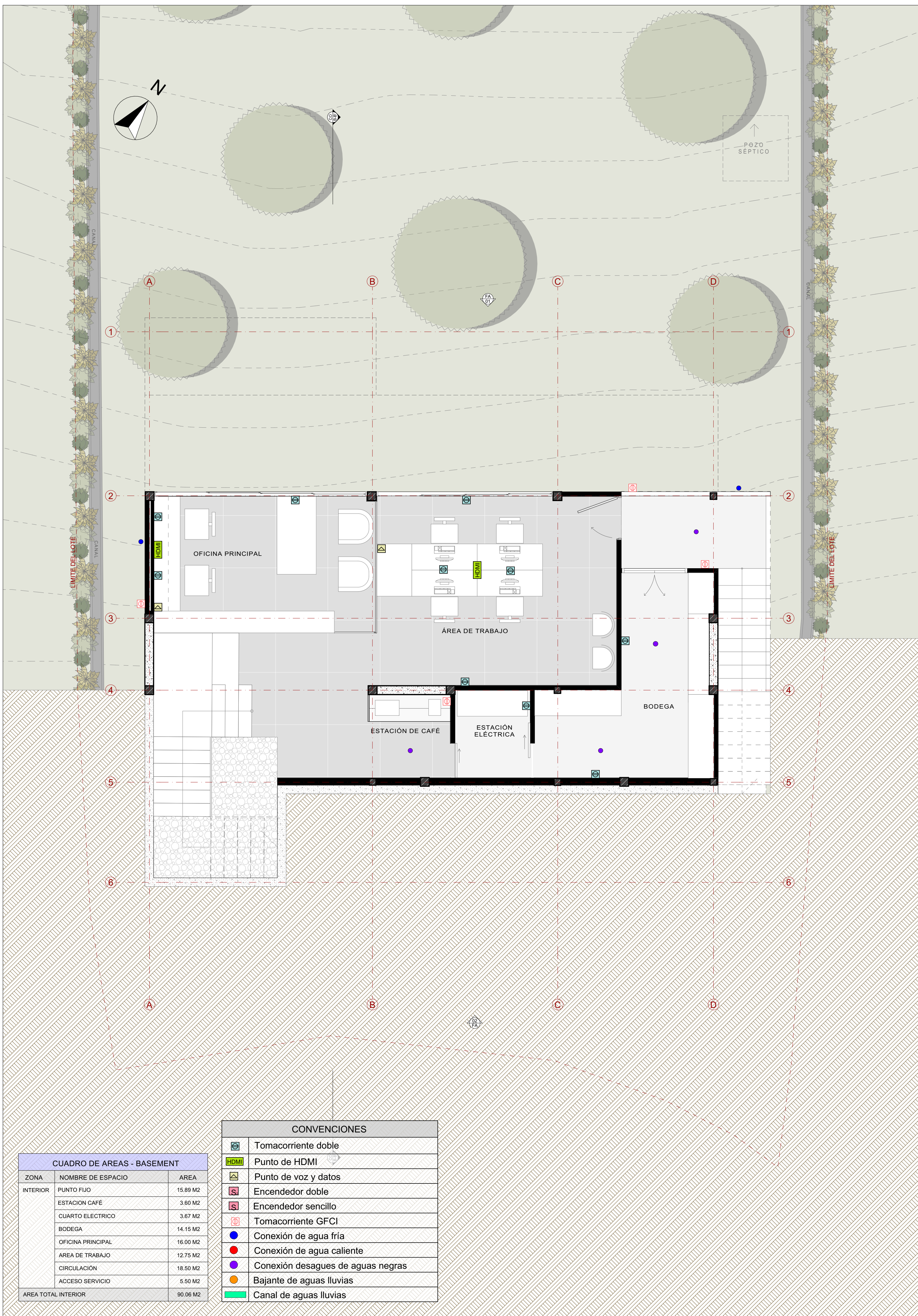
Plano de Sótano:
